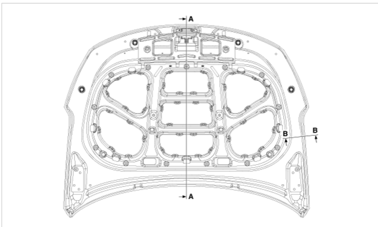
A - A
